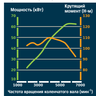
M13A, 4-цилиндровый, DOHC, 1328 см 3
