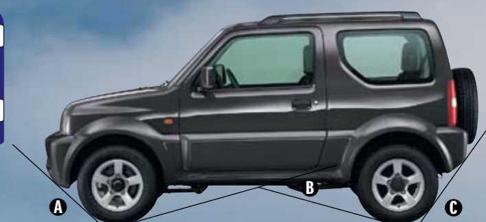
A 37° угол въезда (без груза и пассажиров) B 31° угол рампы C 46° угол съезда
